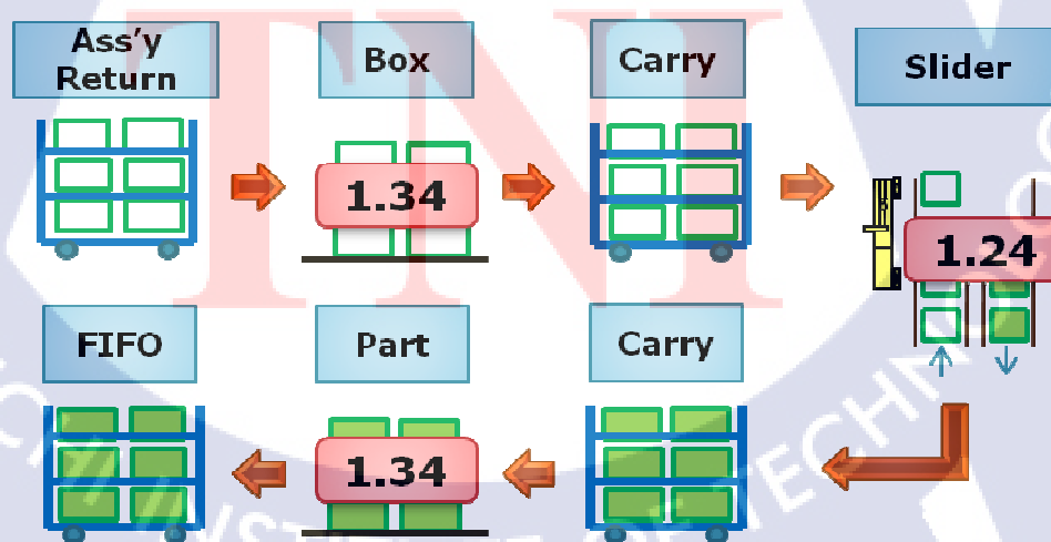
รูปภาพที่ 3.15 แสดงลำดับขั้นตอนของชิ้นงานและเวลาในการยกชิ้นงานขึ้น-ลง
