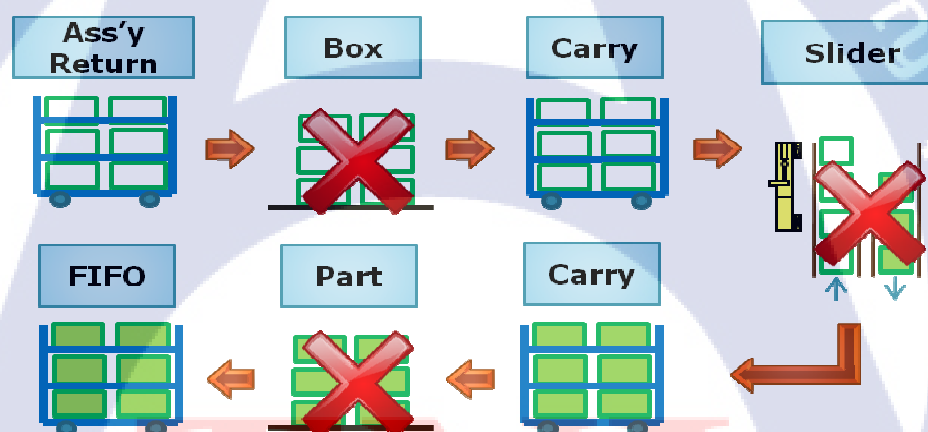
รูปภาพที่ 3.16 ภาพแสดงแนวคิดในการปรับปรุงโดยตัดขั้นตอนการยกชิ้นงานขึ้น-ลง
