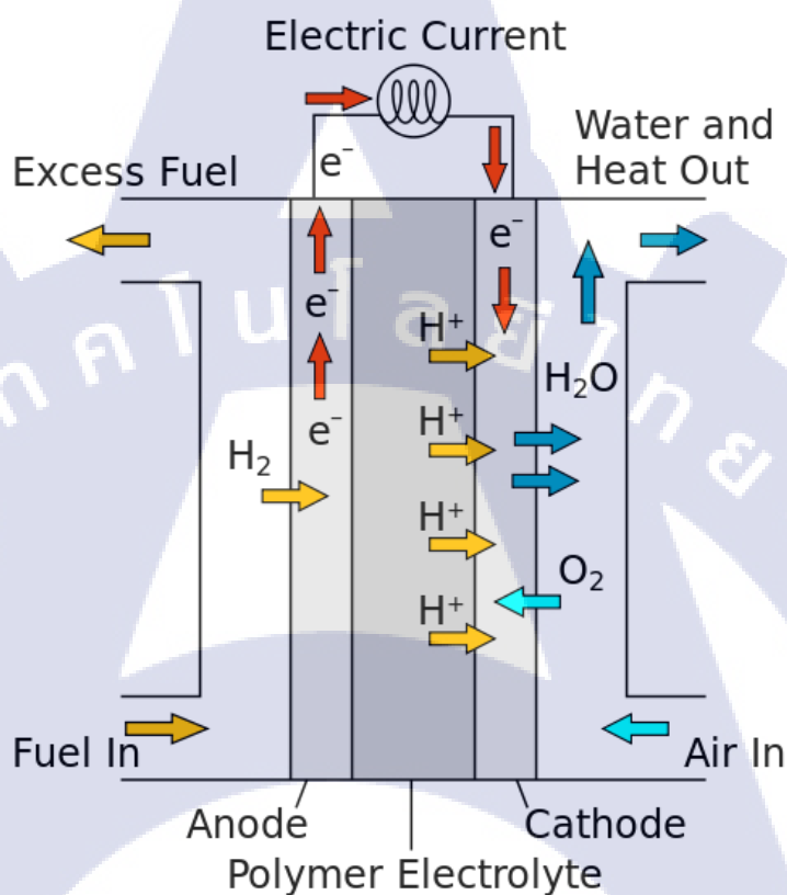
รูปที่ 2.4 การทำงานของเซลล์เชื้อเพลิงแบบพอลิเมอร์อิเล็กโตรไลต์
