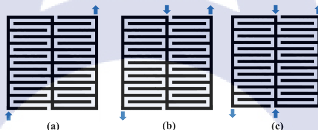
รูปที่ 3. 1แบบจำลอง HIS ที่วิเคราะห์ในโครงการนี้ (a) 1-IO HIS, (b) 1I-2O HIS and (c) 2-IO HIS
