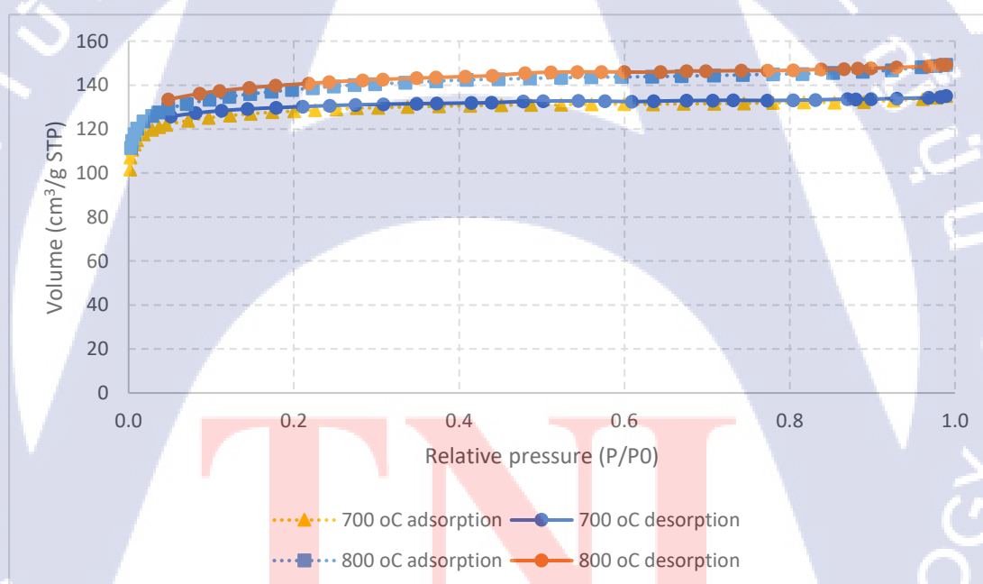
รูปที่ 4.6 Adsorption-desorption isotherm of activated carbon at 700 °C and 800 °C
