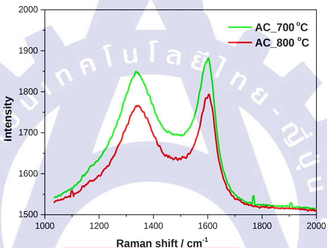
รูปที่ 4.10 Raman spectra activated carbons prepared by calcined at 700 และ 800 °C
