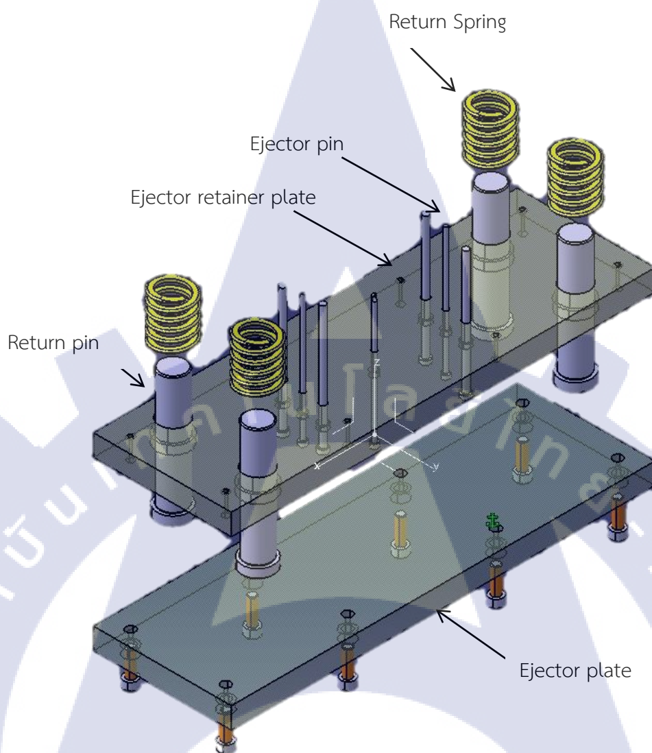
รูปที่ ก.12 ขั้นตอนการประกอบระบบปลดชิ้นงาน (Ejector system)
