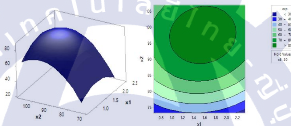
รูปที่ 2.15 รูปพื้นผิวดตอบสนอง (ด้านซ้าย) และเส้นโครงร่าง (ด้านขวา) ของสมการพื้นผิวดตอบสนอง
