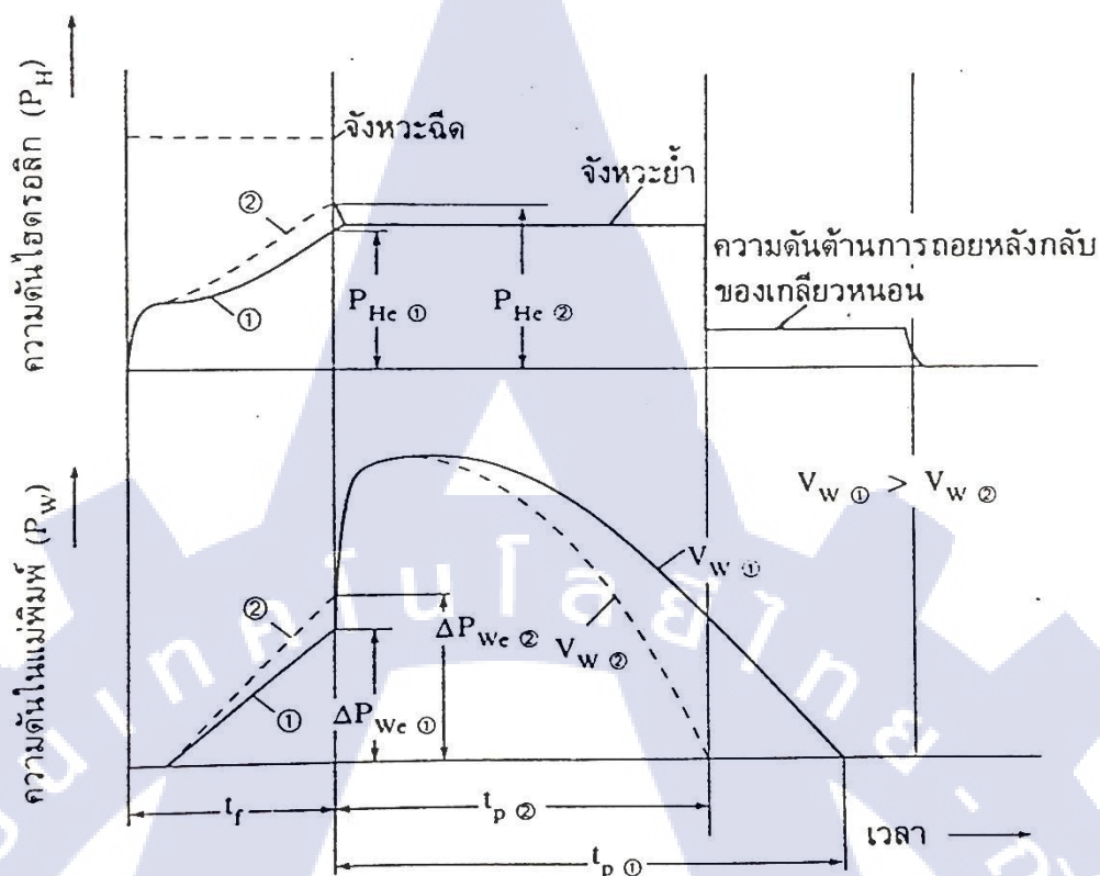
รูปที่ 2.12 อิทธิพลของอุณหภูมิแม่พิมพ์ที่มีต่อความดัน [6]
