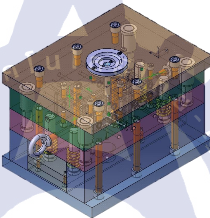
รูปที่ ก.8 แม่พิมพ์ฉีดพลาสติกที่ใช้ในการวิจัย (Assembly mode)
