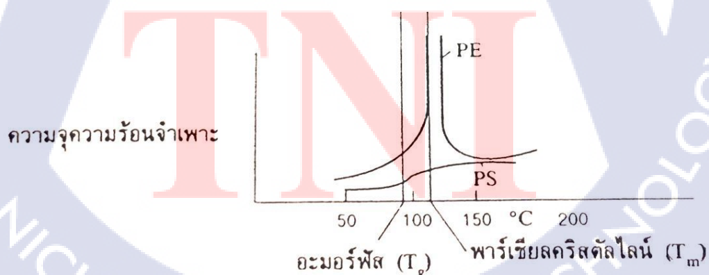
รูปที่ 2.5 ตัวอย่างคุณสมบัติของความจุความร้อนจำเพาะของอะมอร์ฟัสเทอร์โมพลาสติกและพาร์เซิลคริสตัลไลน์เทอร์โมพลาสติก [6]
