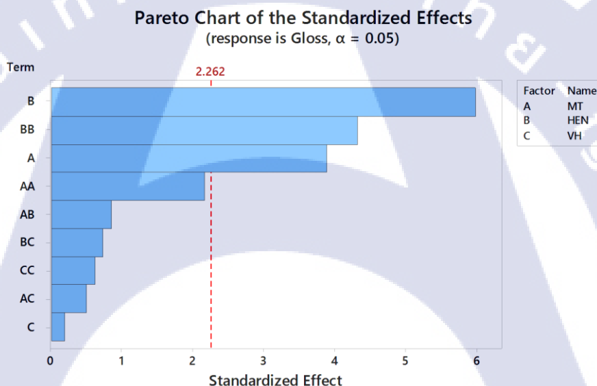
รูปที่ 4.6 แผนภาพพาร์โตแสดงอิทธิพลของตัวแปรที่ศึกษา
