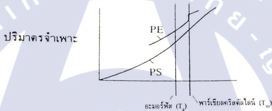
รูปที่ 2.4 ตัวอย่างคุณสมบัติของปริมาตรจำเพาะของอะมอร์ฟัสเทอร์โมพลาสติกและพาร์เซิลคริสตัลไลน์เทอร์โมพลาสติก [6]
