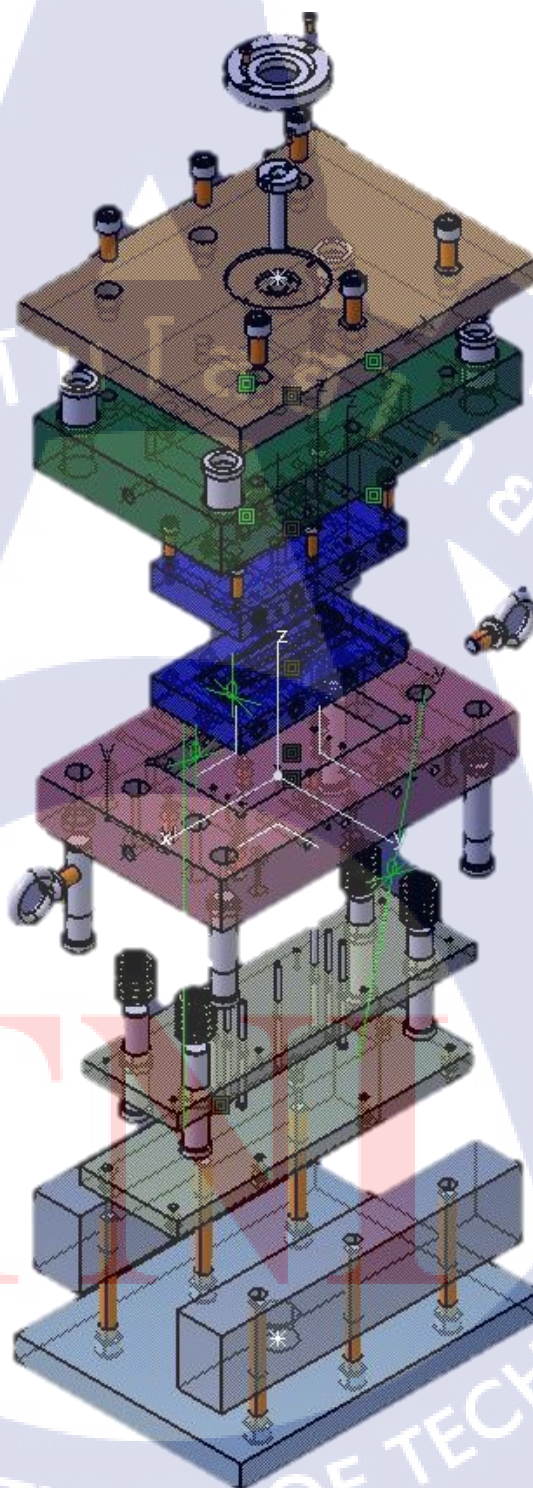
รูปที่ ก.9 แม่พิมพ์ฉีดพลาสติกที่ใช้ในการวิจัย (Explode mode)
