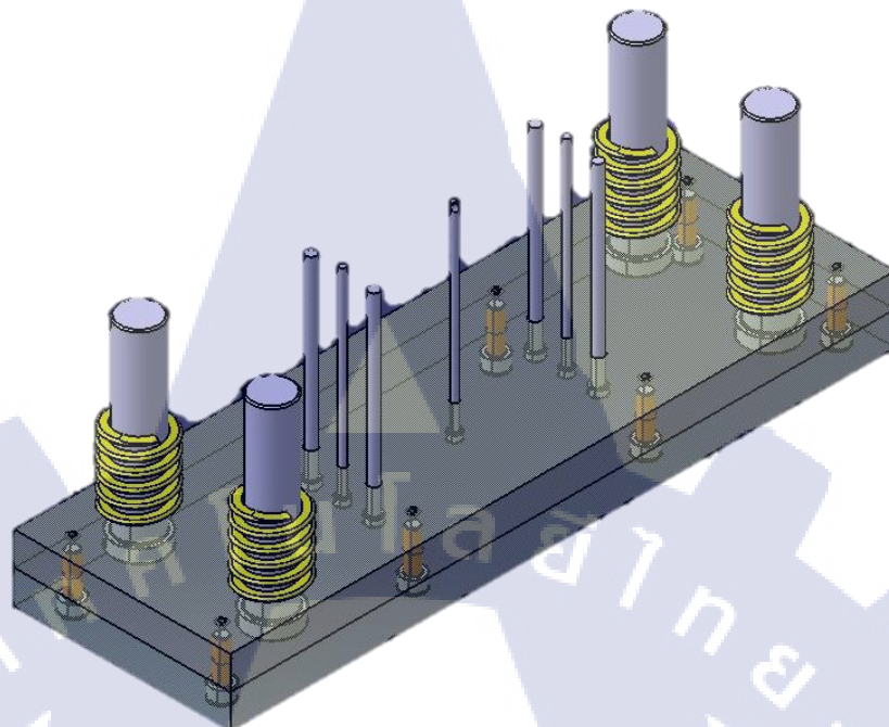
รูปที่ ก.13 ระบบปลดชิ้นงาน (Ejector system)
