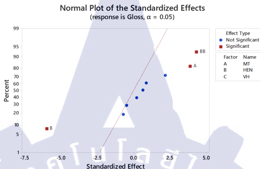
รูปที่ 4.7 แผนภาพปกติแสดงอิทธิพลของตัวแปรอิสระที่ศึกษา
