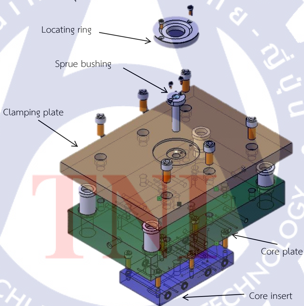
รูปที่ ก.10 ขั้นตอนการประกอบแม่พิมพ์ส่วนอยู่กับที่ (Clamping side)
