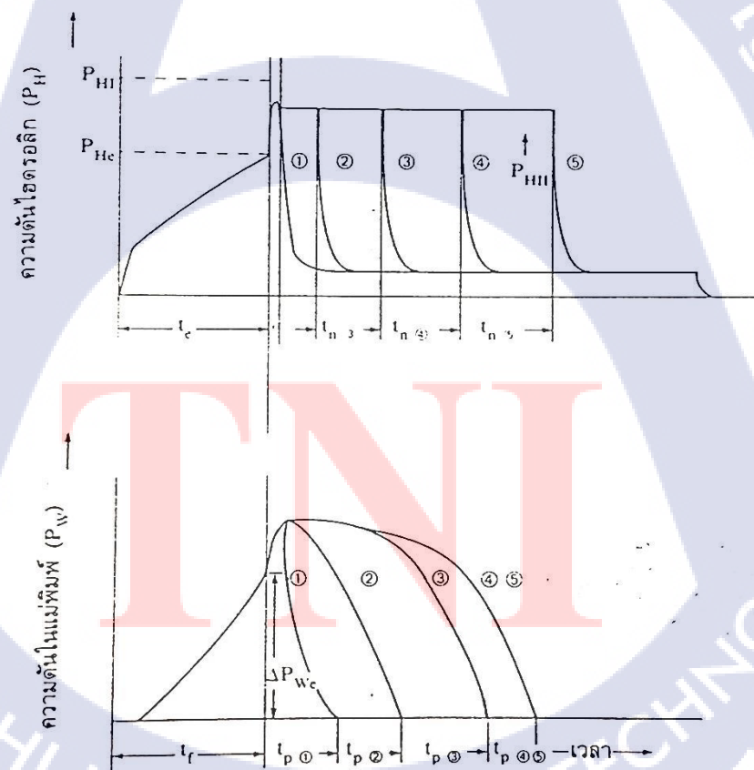
รูปที่ 2.10 อิทธิพลของเวลาในการรักษาคความดัน [6]
