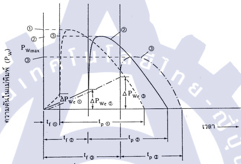
รูปที่ 2.8 อิทธิพลของความเร็วในการฉีด [6]
