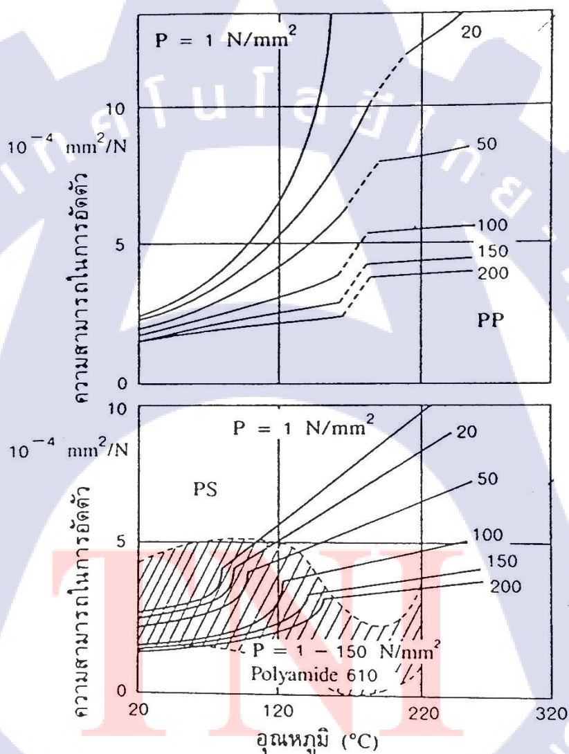
รูปที่ 2.6 ความสามารถในการอัดตัวของพลาสติกเนื่องจากอุณหภูมิและความร้อน [6]
