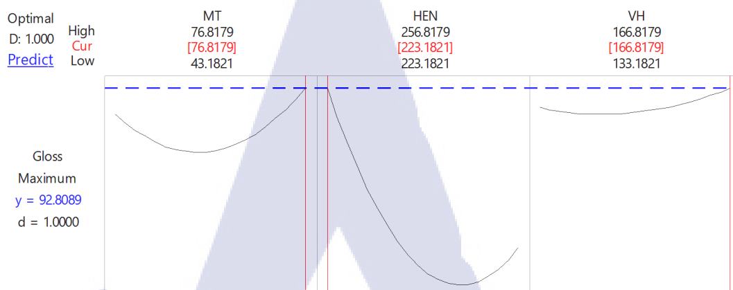
รูปที่ 4.17 แผนภาพแสดงการหาจุดที่มีความมันเงาสูงสุดของตัวแปรทั้งสาม
