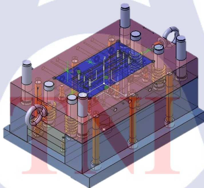
รูปที่ ก.16 แม่พิมพ์ฝั่งเคลื่อนที่ที่ประกอบเสร็จสมบูรณ์
