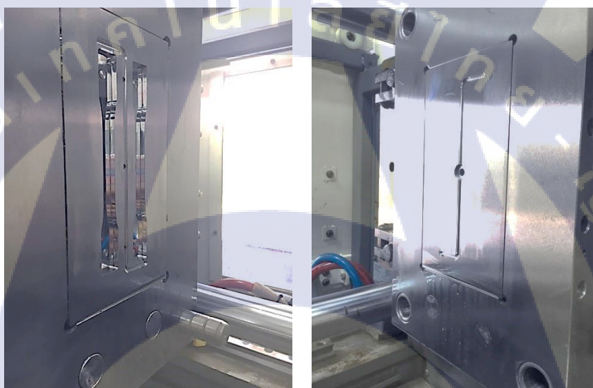
รูปที่ 3.3 แม่พิมพ์ฉีดพลาสติกและแม่พิมพ์อินเสิร์ตฝังควาวิตี (ซ้าย) และคอร์ (ขวา)
