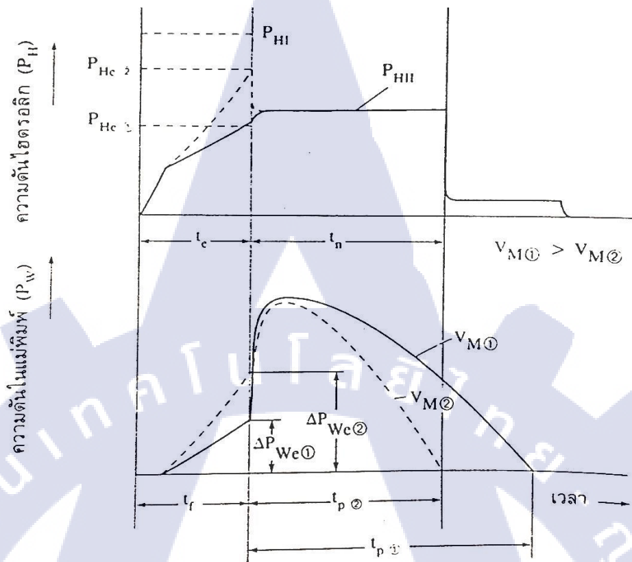
รูปที่ 2.11 อิทธิพลของอุณหภูมิพลาสติกหลอมเหลวที่มีต่อความดันในแม่พิมพ์ [6]
