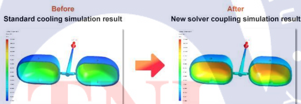
รูปที่ 2.17 การจำลองการไหลของพลาสติกในโปรแกรม Moldex3D R14 [9]
