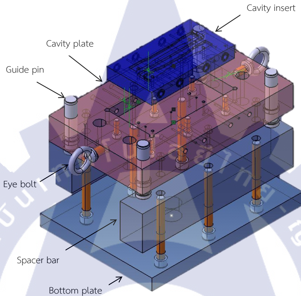
รูปที่ ก.14 ขั้นตอนการประกอบแม่พิมพ์ส่วนเคลื่อนที่ (Moveable side)
