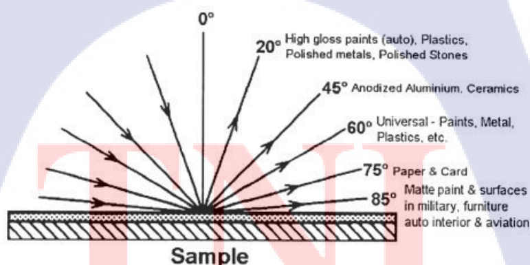
รูปที่ 2.14 มุมที่ใช้วัดความเงา (Gloss angle) [7]
