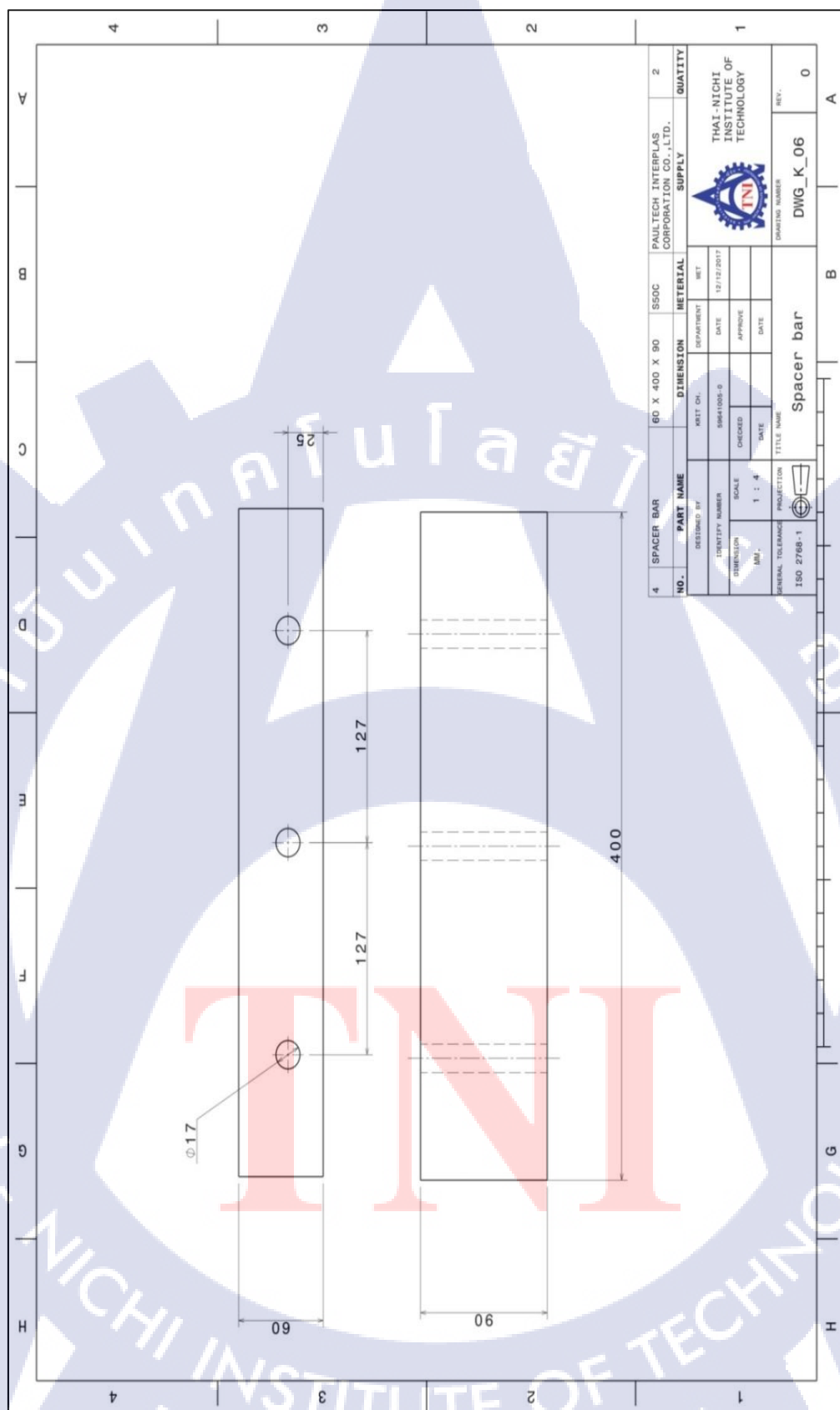
รูปที่ ข.7 ภาพแยกชิ้นของแม่พิมพ์ฉีดพลาสติกชิ้นส่วนหมอนรองแม่พิมพ์
